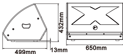
HV8(N)全频音箱
