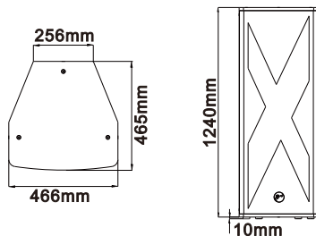
HV215(N)全频音箱
