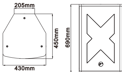
HV15(N)全频音箱
